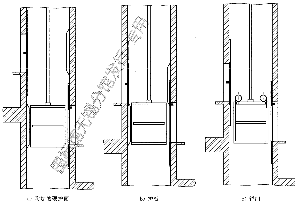
图 F.1 防止货物碰撞的保护措施
