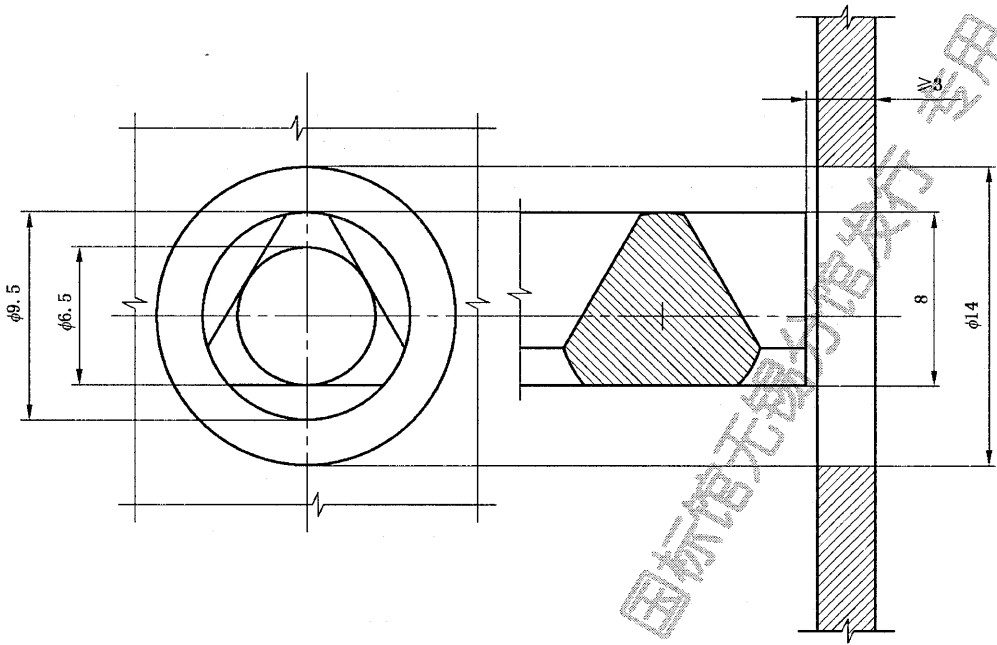
图 B.1 开锁三角形钥匙
