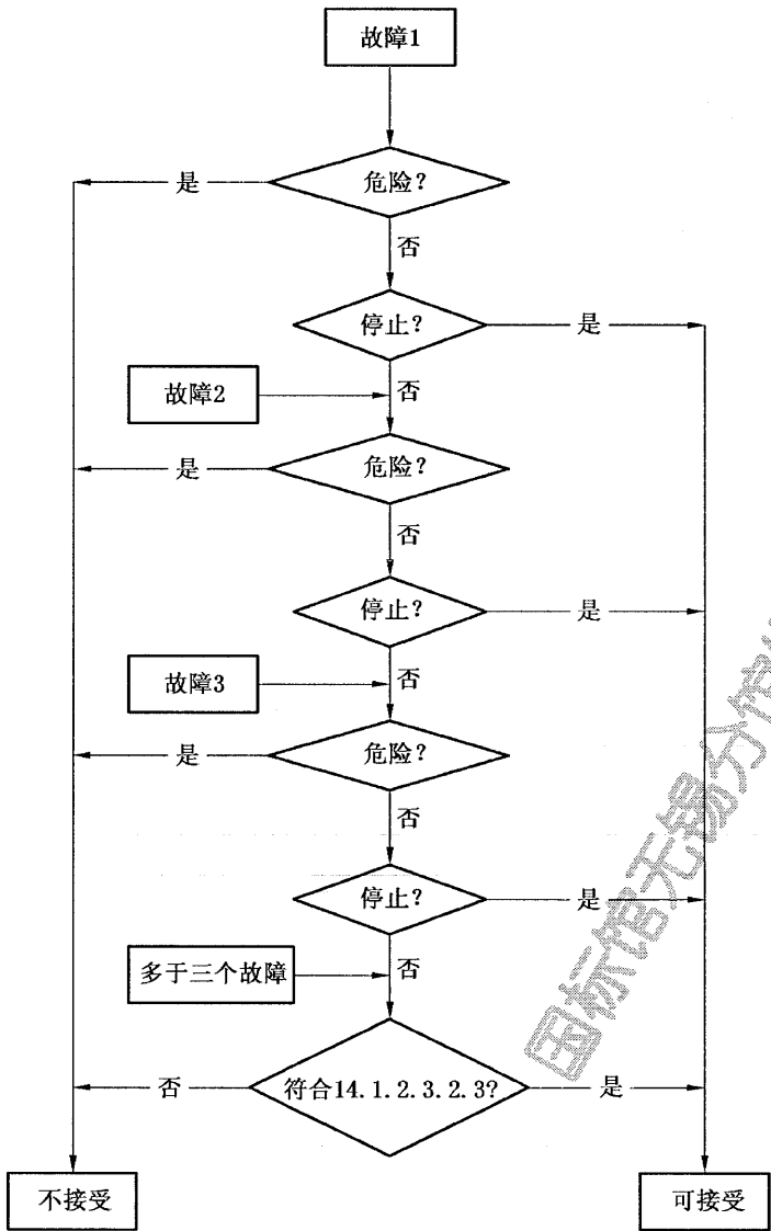
图 1 安全电路评价流程图
